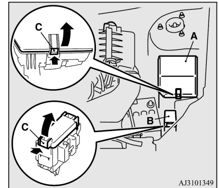
A - 主保險絲盒 B - 副保險絲盒
